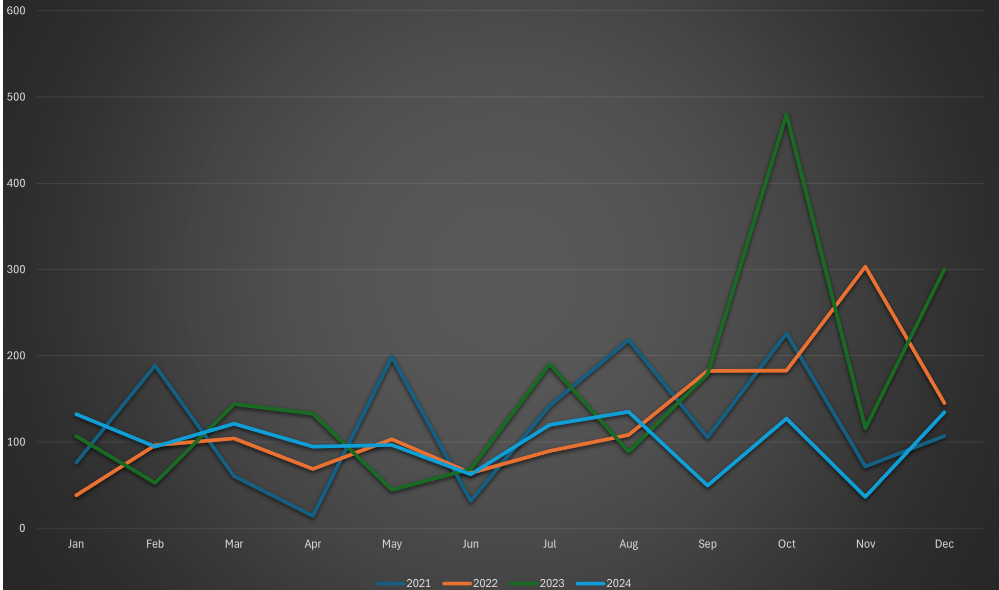
2021-2024 Rain mm
